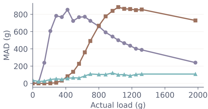
(d) Median absolute deviation
